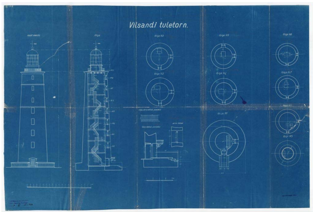
Joonis 20. Väljavõte Vilsandi tule torni ülesmõõtmisjoonistest 1925. aastast, kui täiustati tule torni valgussüsteemi. Eesti Meremuuseum 2396:161 D 537:161.
