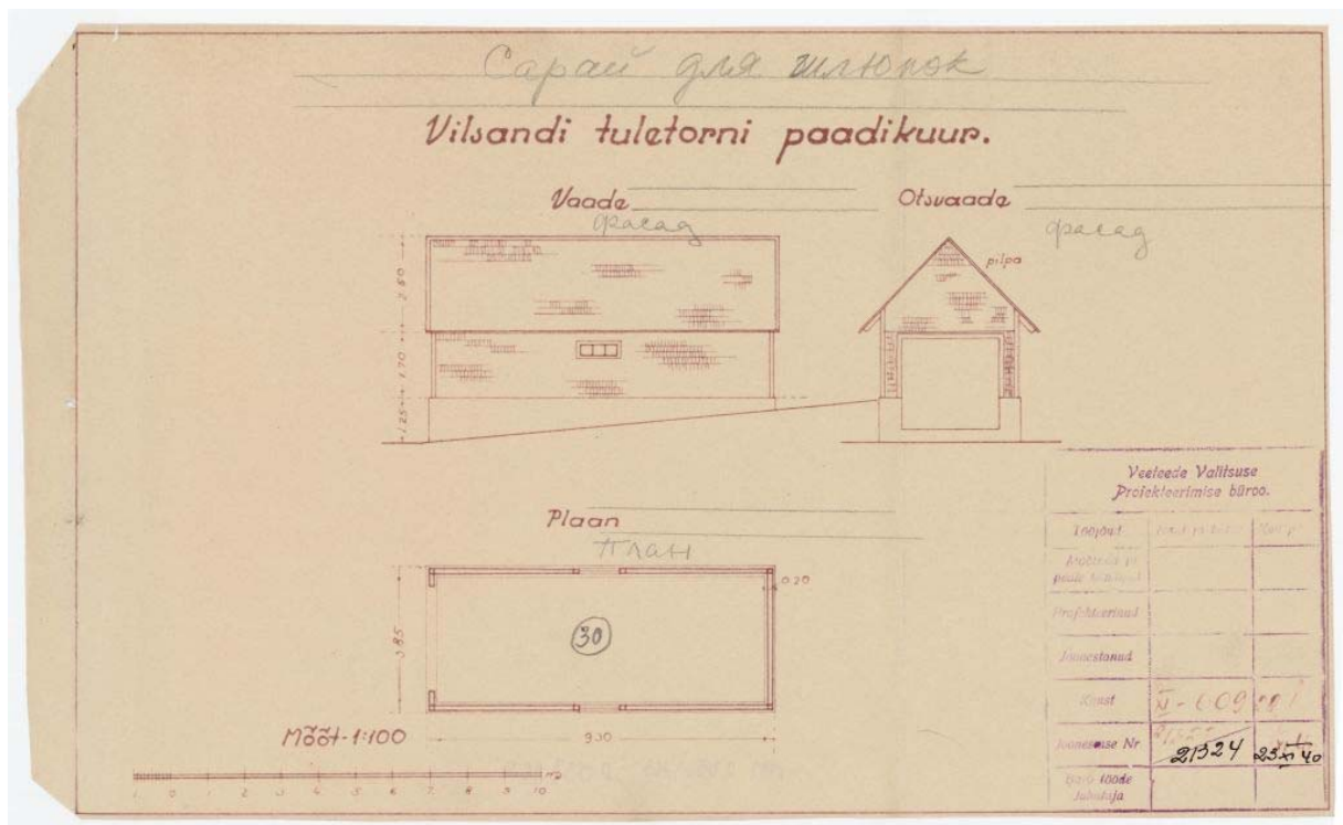
Joonis 21. Vilsandi tule torni paadikuuri ülesmõõtmisjoonis 1910. aastast. Eesti Meremuuseum 2396:168 D 537:168.
